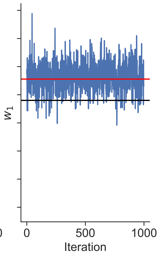
Posterior distributions Dataset 37
