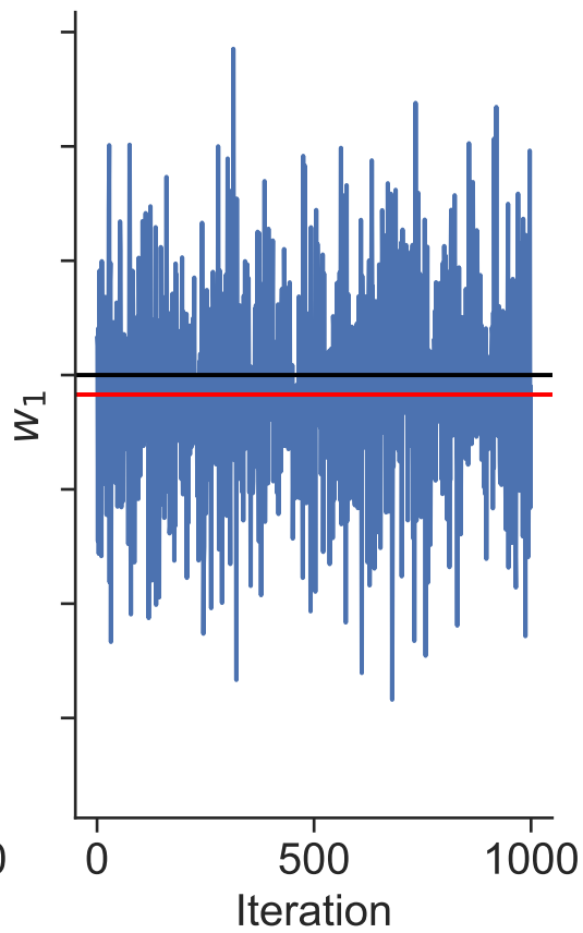
Posterior distributions Dataset 10
