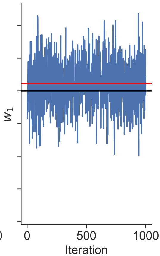
Posterior distributions Dataset 42
