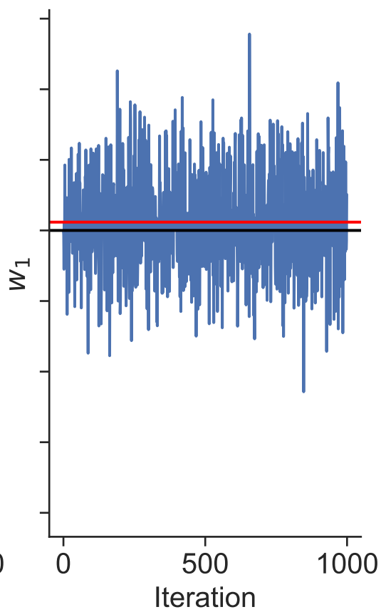
Posterior distributions Dataset 27
